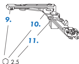
Rækkefølge ved fastklemning (eksempel: hængselside foroven)
