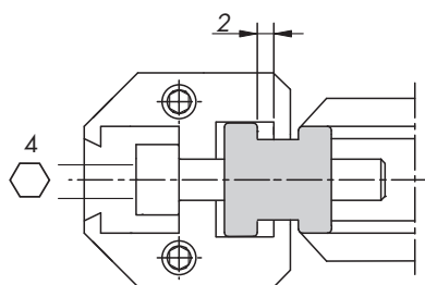
Grundposition justeringsstykke med 2 mm spaltmål
