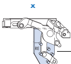
Montering af lære og visninger af hjørnelejer (eksempel: hængselside forneden)
